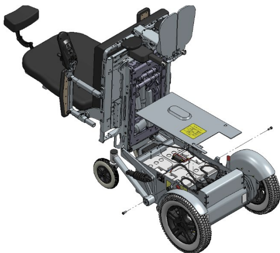
Afbeelding 3 Open de stoel voor de batterijruimte
