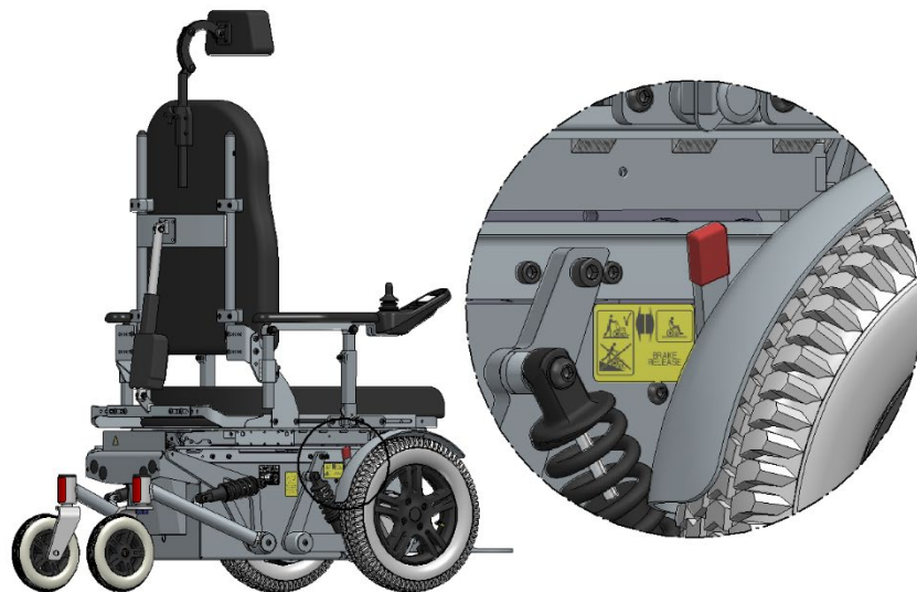
Afbeelding 9 De rolstoel in de rijfunctie
