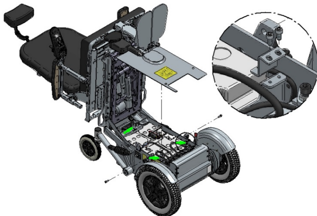
Afbeelding 6 Vervanging van de batterij
